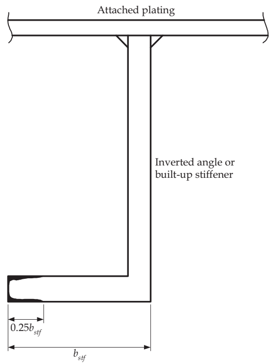
Fig. 12.1.2 Edge Corrosion
