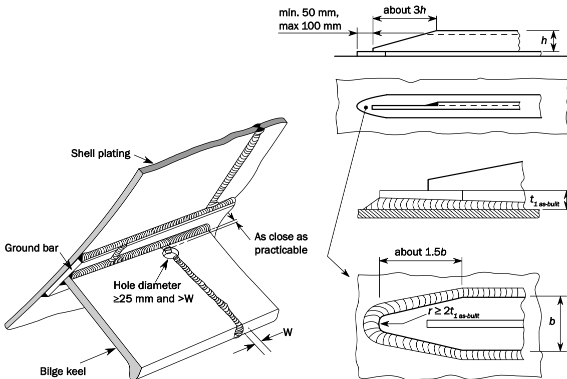
Fig. 10 Bilge keel
