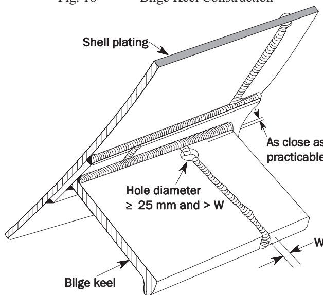
Fig. 18 Bilge Keel Construction
