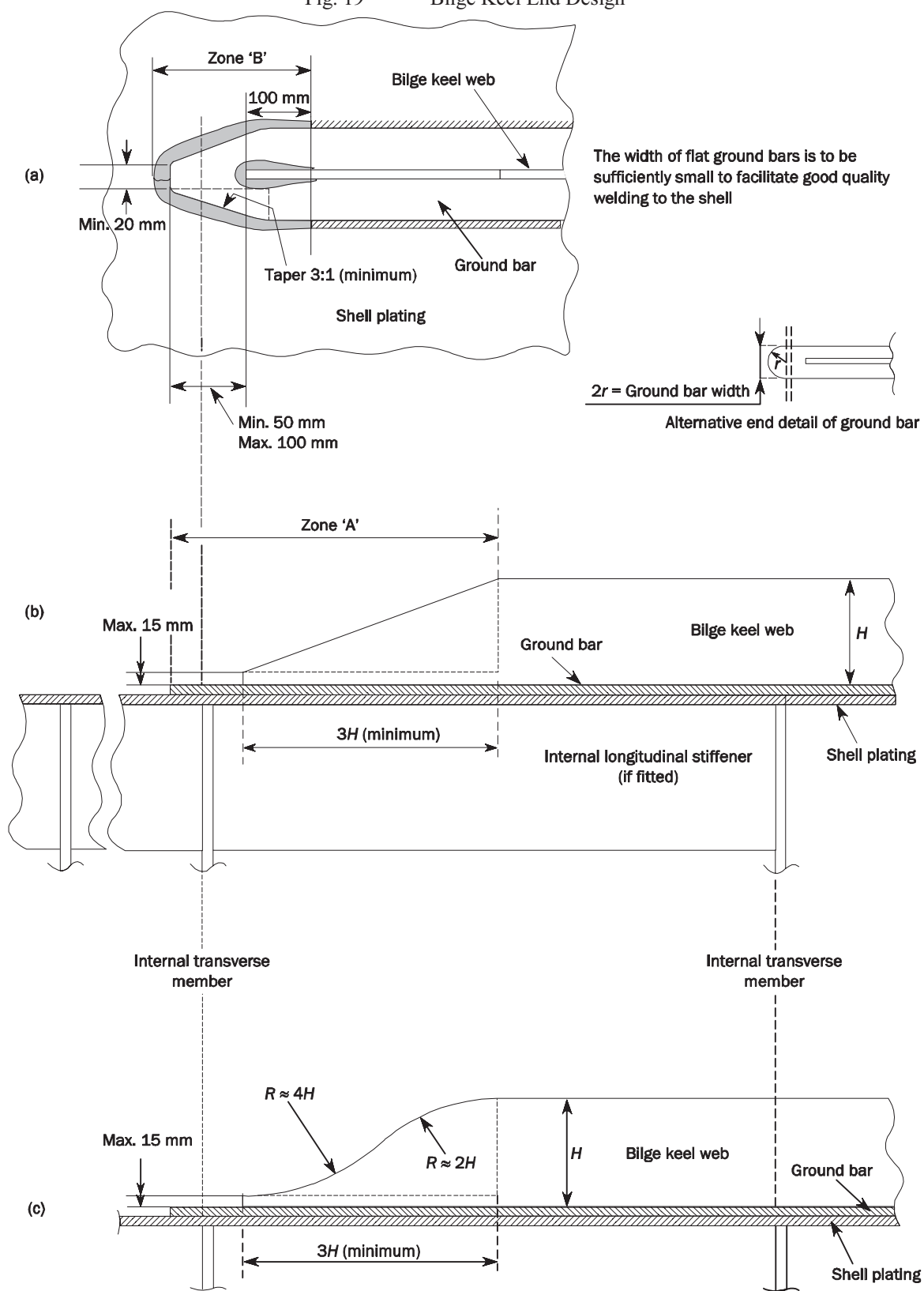
Fig. 19 Bilge Keel End Design
