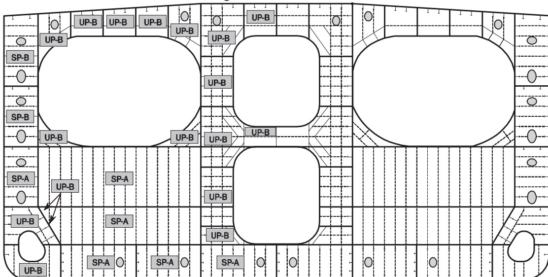
Fig. 4 Cross Tie
