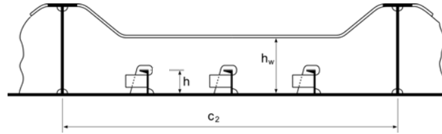
Figure 5 - Parameter Definition for Web Stiffening
