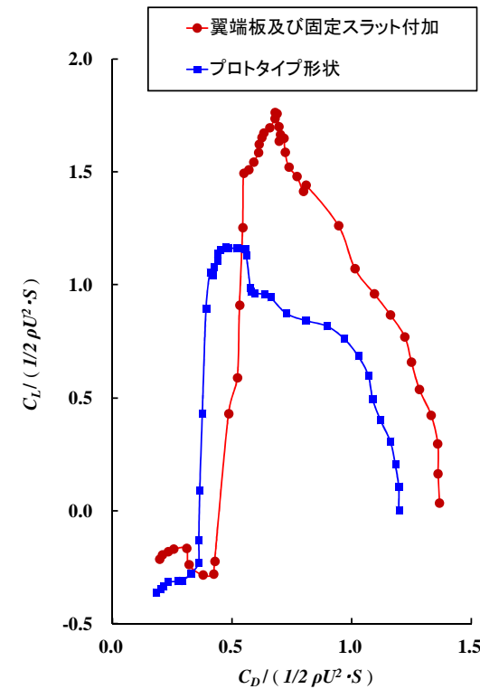
空力特性
