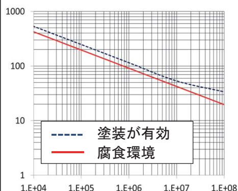
CSRのS-N線図
