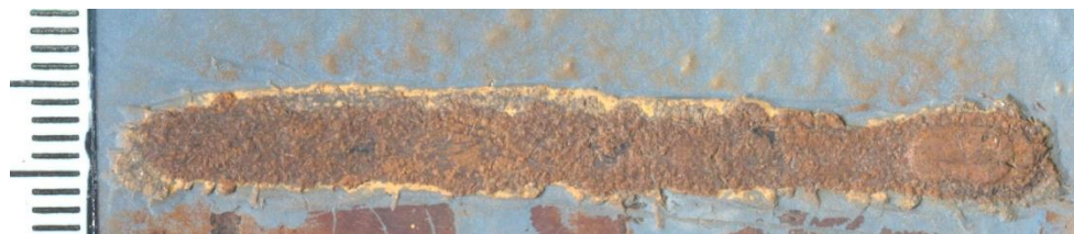
図 C-6 ウェーブタンク試験の側面試験片におけるスクライプからのさび幅（冷却あり）（このモデル報告書の結果例は写真例と関係ない）
