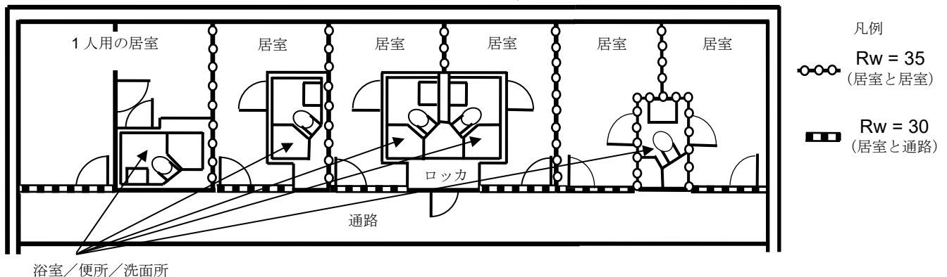
図 An5.1.1 居室の配置例
