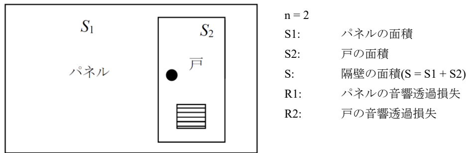
図 An5.1.2 隔壁を構成する遮音パネル及び戸
