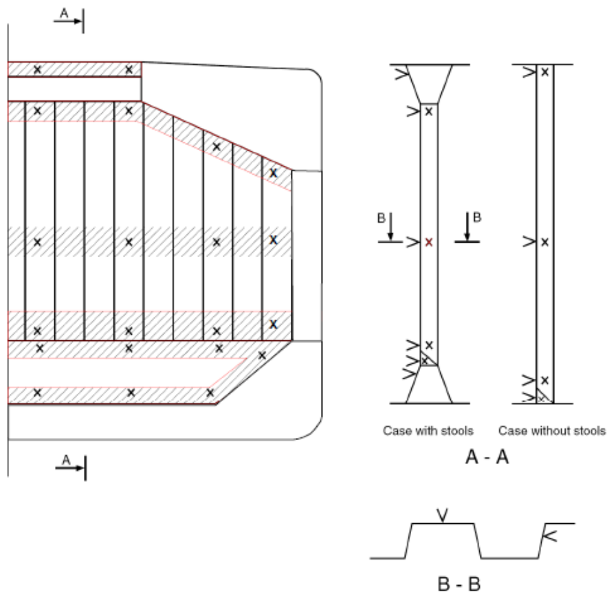
二重船側構造ばら積貨物船
