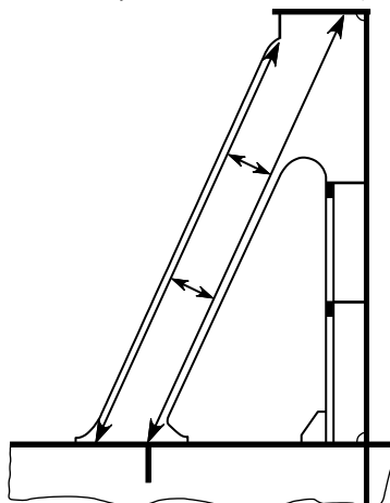
図 8 ハッチコーミングステイ (例 3)
