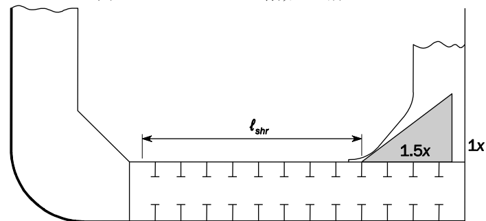
図 2 フロアの有効せん断スパン
