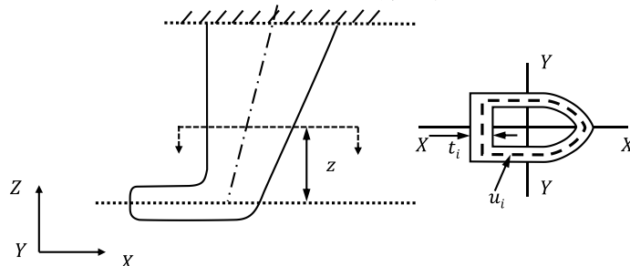
図 CS3.4.1-6. ラダーホーン薄肉部の断面
