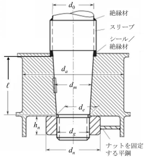
図 CS3.8 キー付コーンカップリング
