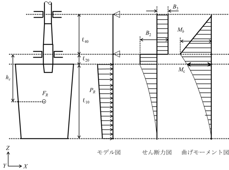
図 CS3.4.1-3. C型舵
