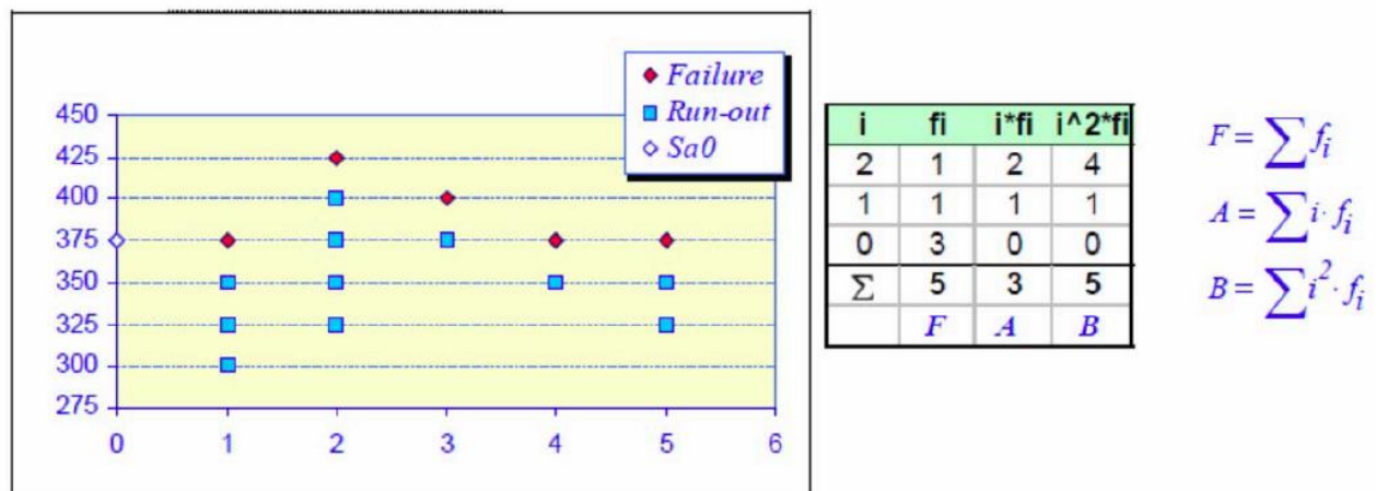
図 2 修正ステアケース法の試験結果の処理方法
