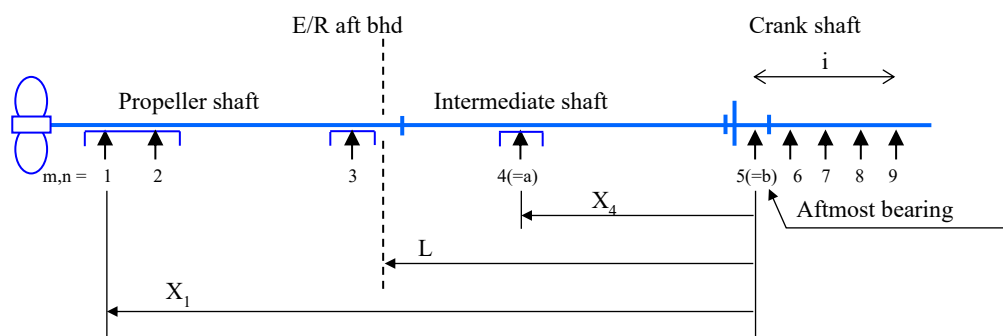
図 1.3.3-1.(b) 軸受番号及び支点番号
