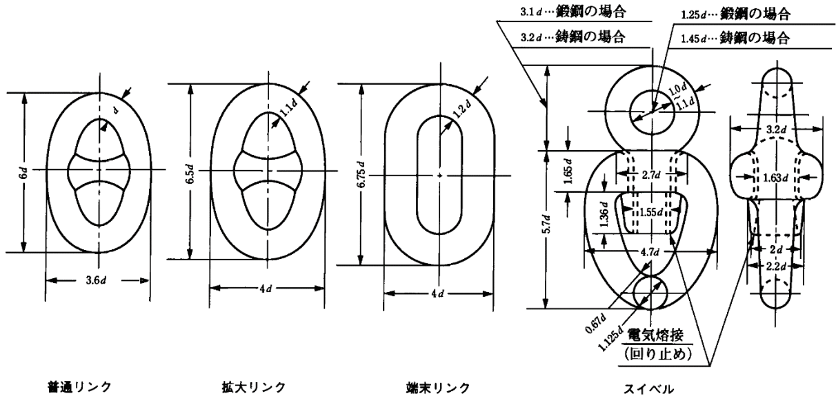
(1) スタッドなしチェーン
