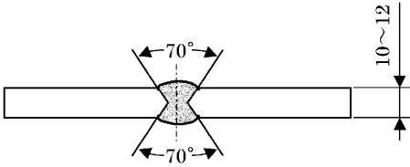
両面溶接の場合
