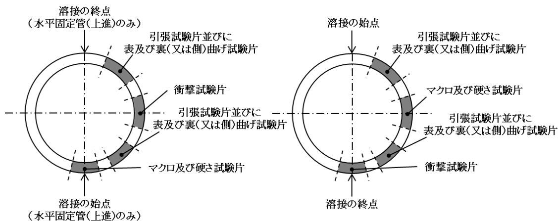
(B)管の試験材 ((C)に示す溶接姿勢を除く) (C)管の試験材 (水平固定管 (下進) の場合)
