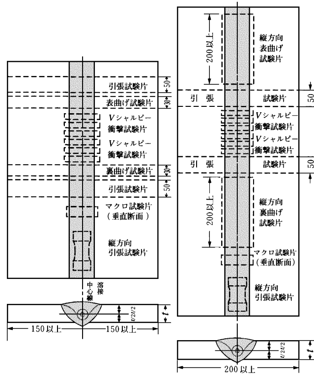
(a) (b) 以外の試験材 (b) KAWL 91, KAWL 92 用試験材
