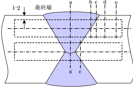
(d) 両面溶接の場合 (厚さ 50 \text{ mm} 超え)
