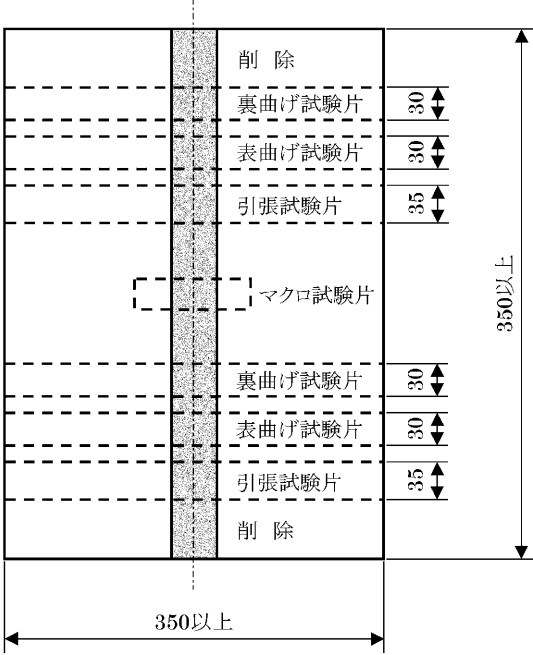
図 M6.20 突合せ溶接試験材 (板厚 30~12mm の場合, 単位 mm)
