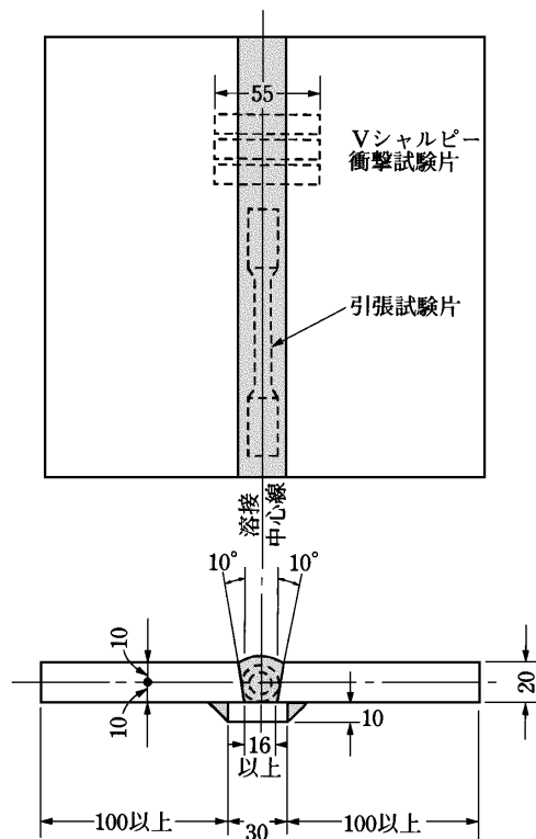
図 M6.1 溶着金属試験材 (単位 mm)
