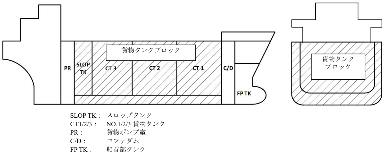
図 R4.5.1-5. 貨物タンクブロックの例
