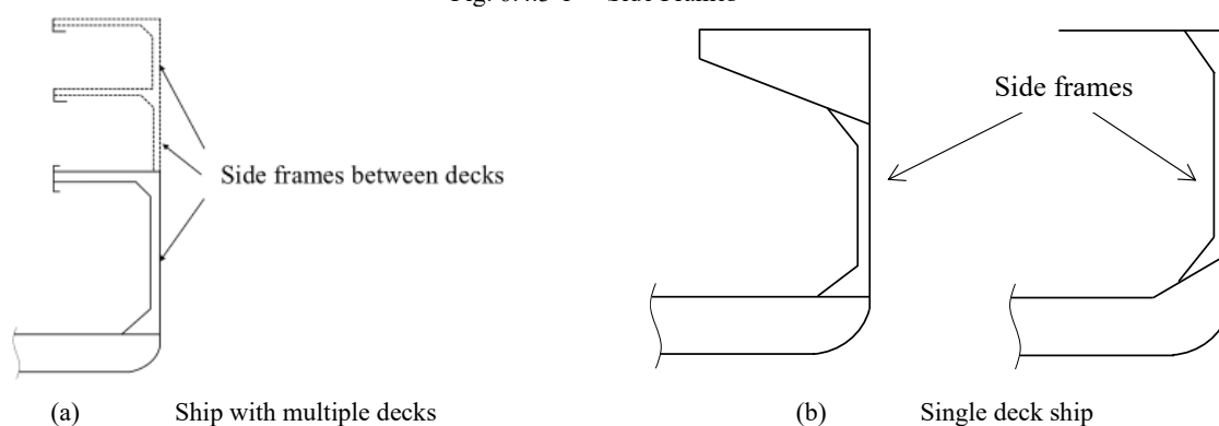
Fig. 6.4.3-1 Side Frames
