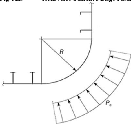
Fig. An9 Transverse Stiffened Bilge Plating
