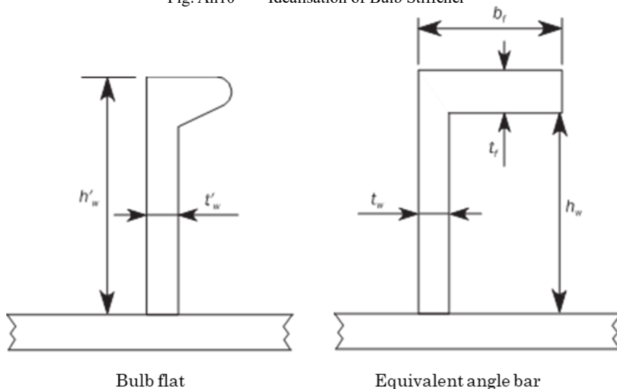
Fig. An10 Idealisation of Bulb Stiffener
