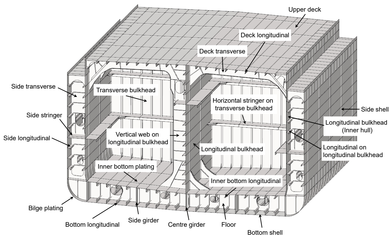
Fig. 1.4.5-8 Tanker
