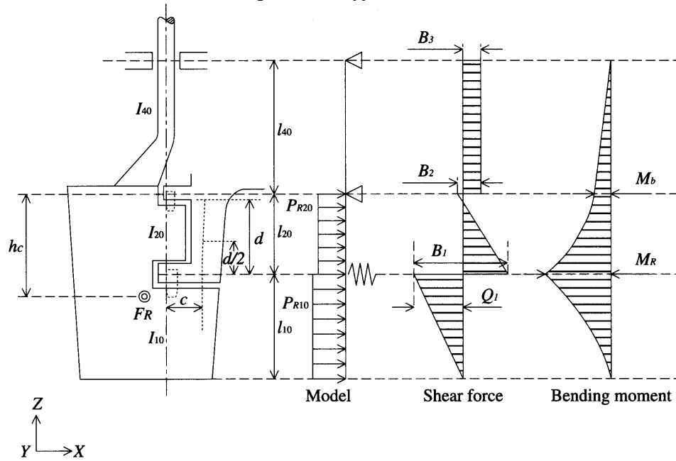
Fig. C3.4.1-5 Type E Rudder
