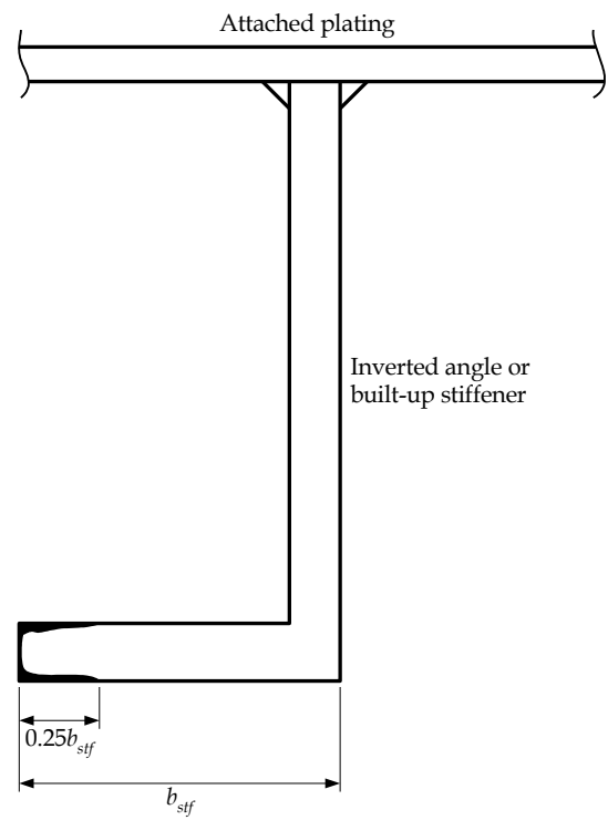
Fig. 12.1.2 Edge Corrosion
