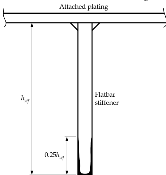
Fig. 12.1.2 Edge Corrosion
