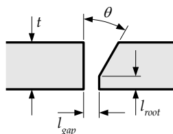
Double bevel butt
