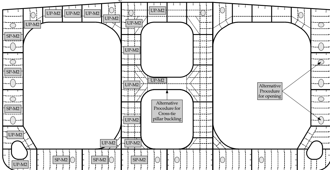
Fig. D.5.2 Transverse Web Frames
