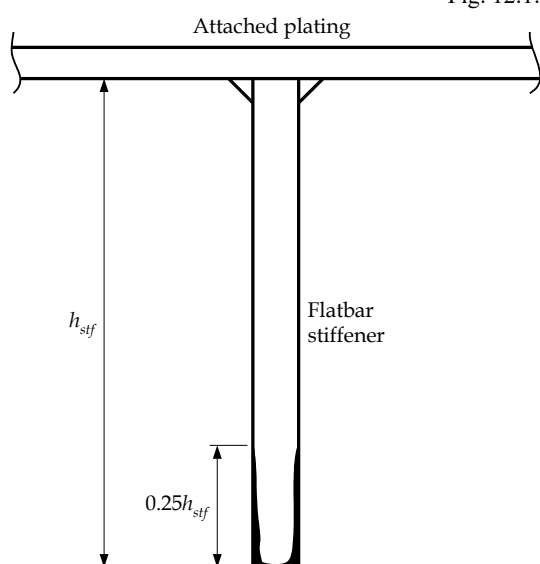
Fig. 12.1.2 Edge Corrosion
