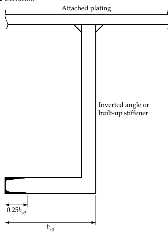
Fig. 12.1.2 Edge Corrosion
