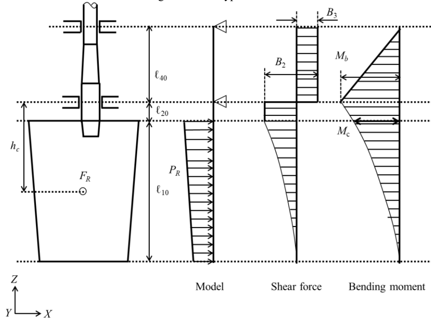
Fig. CS3.4.1-3 Type C Rudder
