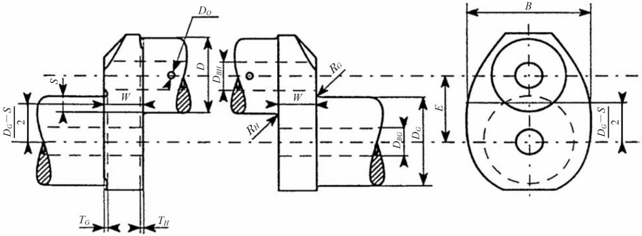
Fig. 5 Crank Dimensions
