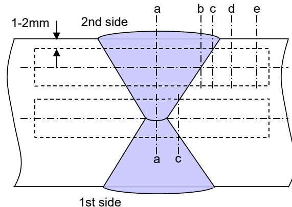
(d) For Both side ( t > 50 mm)
