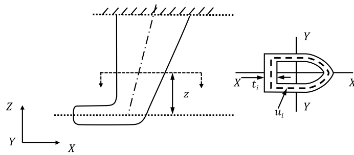
Fig. 4.2.1.6-1 Type A Rudder
