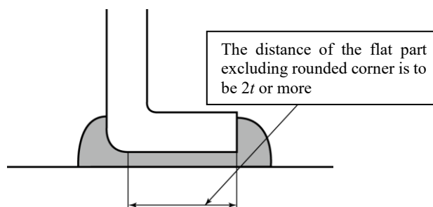
(d) Enlarged View of Rounded Corner
