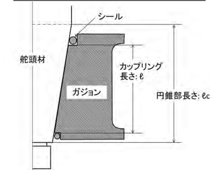
図 CS3.9 円錐部の長さとかップリング長さ
