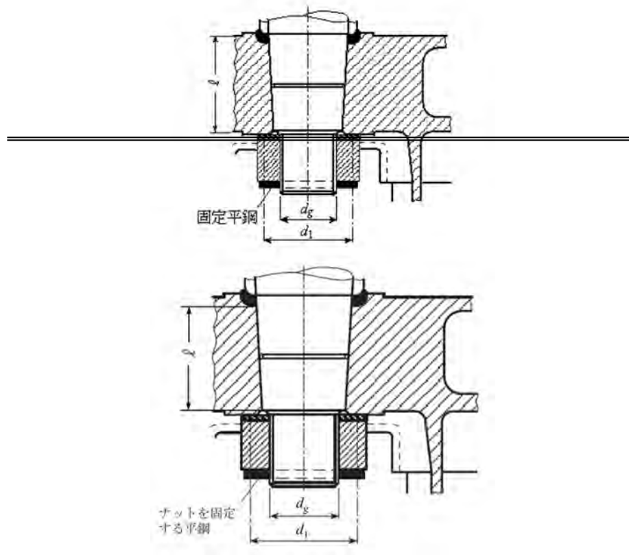
図 CS3.10 キー無しコーンカップリング
