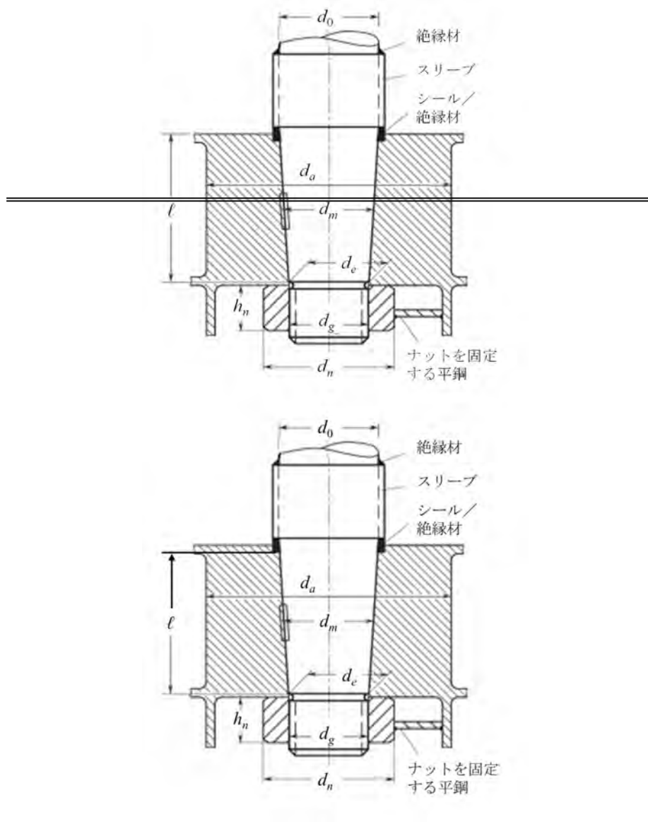
図 CS3.7 キー付コーンカップリング
