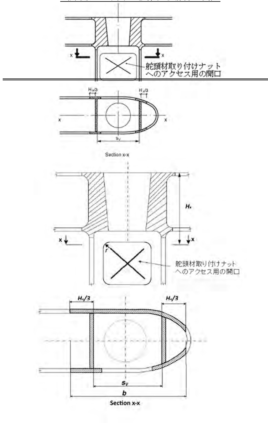
図 CS3.5 舵板構造と舵頭材ハウジング部との接合部横断面 (片側にのみ開口を有する場合の例)
