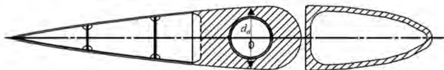
図 CS3.8 ガジヨン外径
