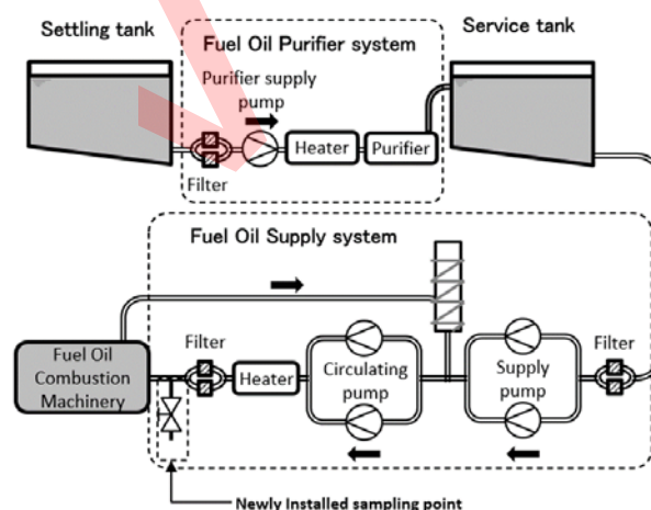
サンプリングポイント設置(改造)例
